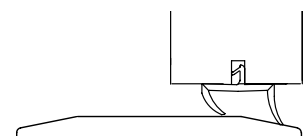
Falsad tröskelplatta med släplis Denna variant finns ej till fanérad karm i Expressortimentet.
